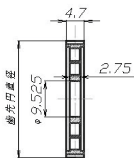
マシンカット (品番: SM6400) DD用スーパーデフ (品番: SR6400)
