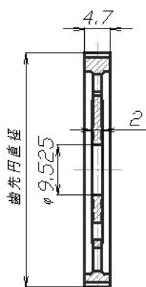
TC用 (品番: ST6400)
