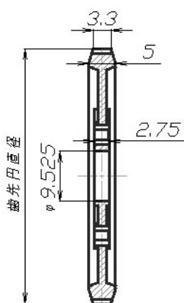
汎用スーパータフ (品番: S6400T・S4800T)
